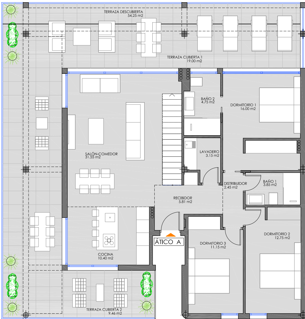
PLANTA ÁTICO
