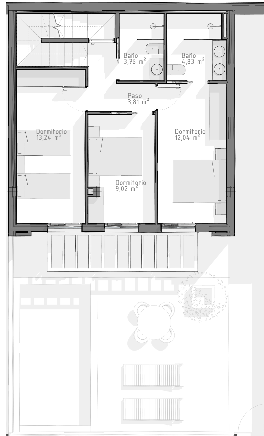
6.Viv. Unifamiliar. Planta 1ª
