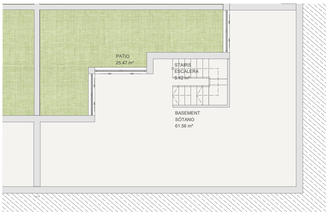
PLANTA SÓTANO
