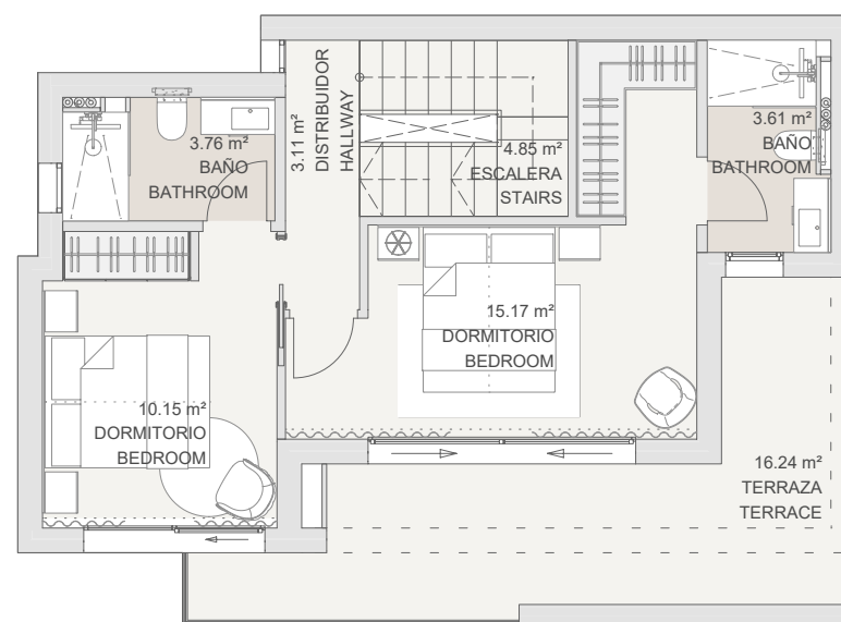
PLANTA PRIMERA
