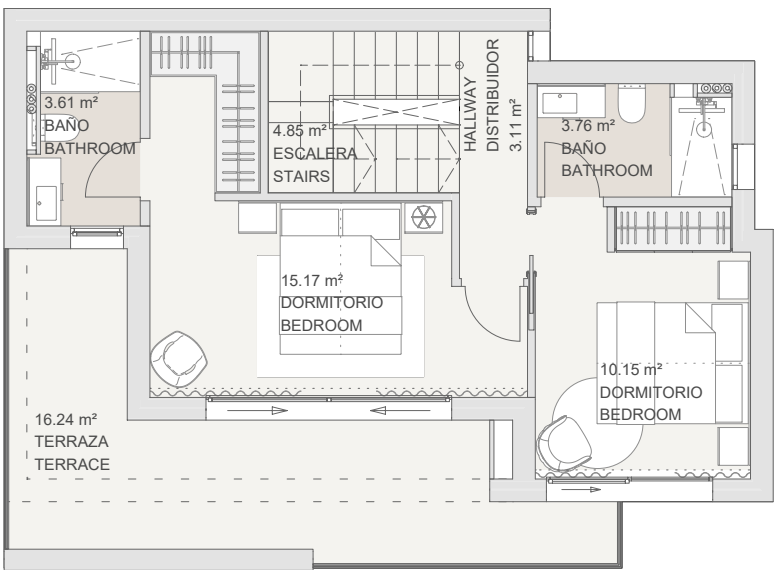
PLANTA PRIMERA
