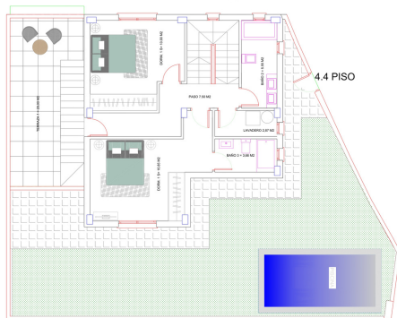
4.4 PLANTA PISO
